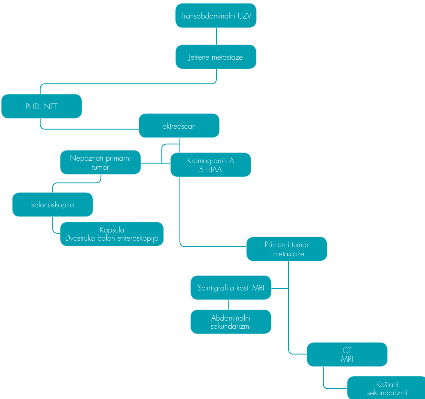
Slika 2.: Dijagnostički algoritam
